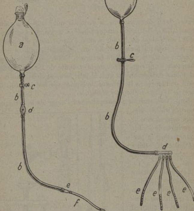
Fig. 29. — Appareil à instillation intermittente. — a . Ampoule d'un litre. — b . Tube irrigateur d'un diamètre de 7 mm. — c . Pince de Mohr. — d . Tube distributeur à 4 branches. — e . Tubes adducteurs (fig. 18).
